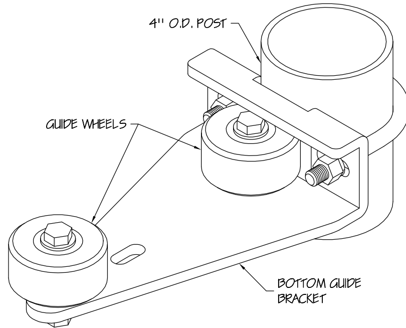
2 BOTTOM GUIDE ASSEMBLY HDC-2 Scale: None
